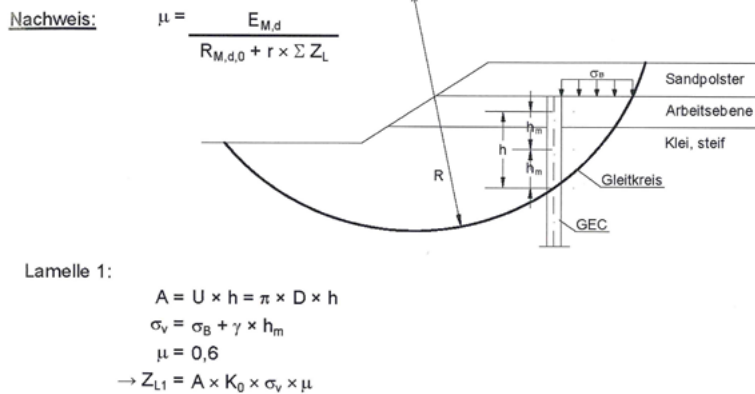
Bild 14. Berechnungsmodell der globalen Sicherheit unter Einbeziehung der „vertikalen“ Bemessungsfestigkeit der geotextilen Ummantelung Fig. 14. Calculation model for the global stability under consideration of the “vertical” design strength of the geotextile encasement
