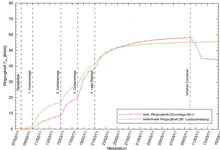
Bild 8. Zeit- und lastabhängige Entwicklung der Ringzugkräfte Fig. 8. Time- and surcharge-dependent development of ring tensile forces
