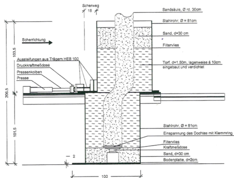
Bild 12. Modellscherversuche an einer ummantelten Säule Fig. 12. Model shear tests on a geotextile encased column
