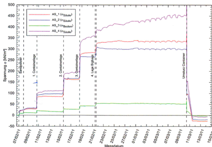
Bild 9. Vertikale Spannungen Fig. 9. Vertical stresses
