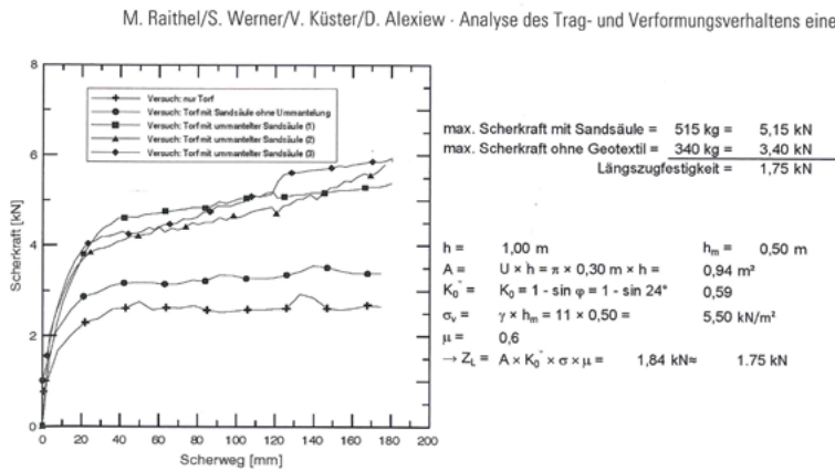
Bild 13. Ergebnisse der Scher-Modellversuche und Vergleichsberechnung Fig. 13. Results of the model shear test and comparative calculation
