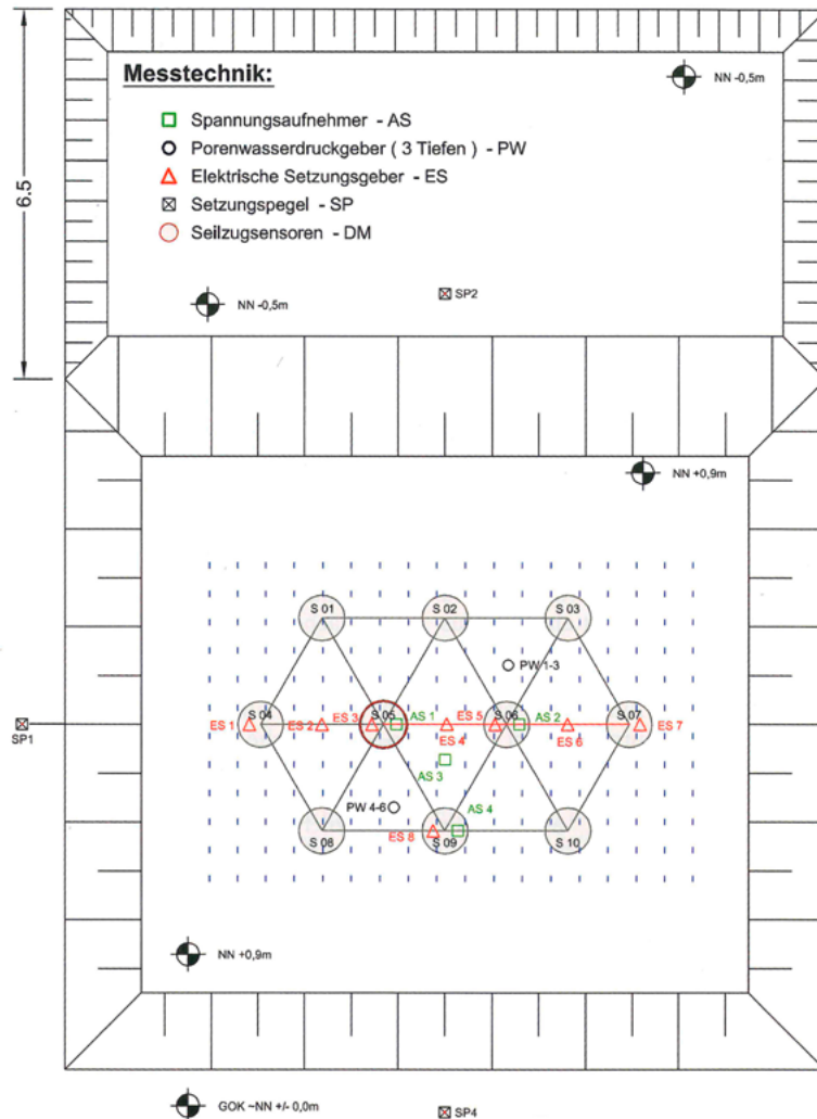
Bild 3. Messstellenplan
